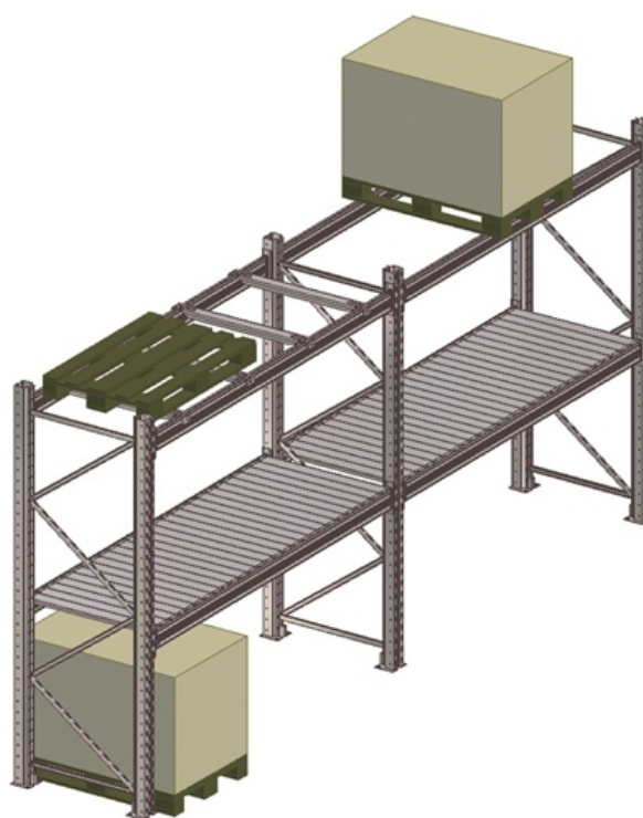
CAMPATE TIPO CON ACCESSORI
